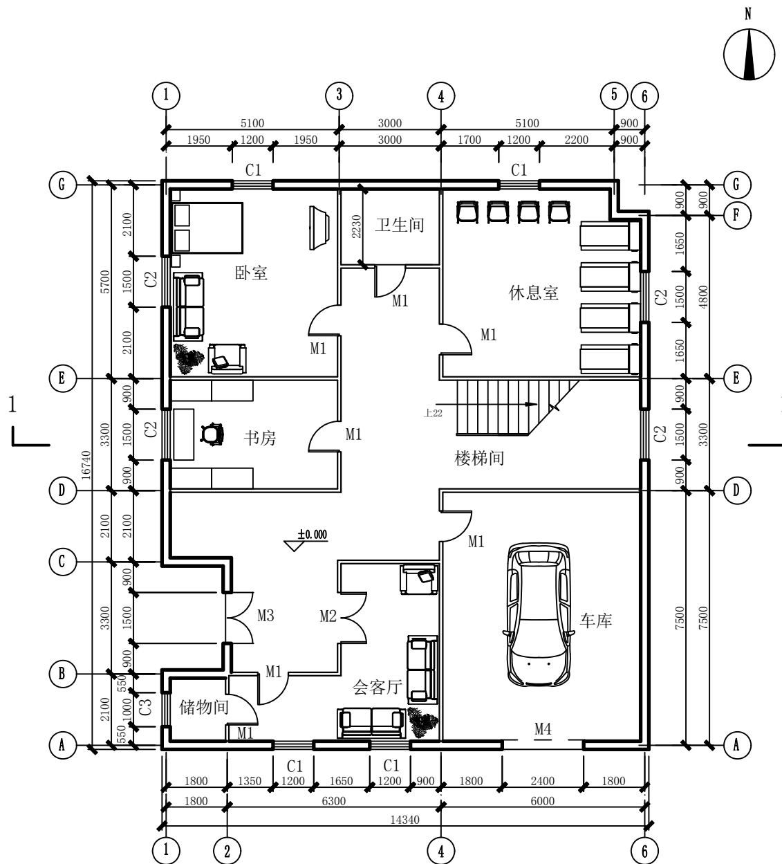
首层平面图 1:100
